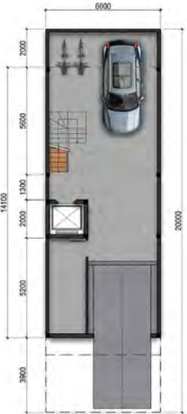
Mặt Bằng Tầng Hầm | Basement Floor
